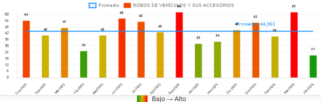
Evolución Mensual de ROBOS DE VEHÍCULOS Y SUS ACCESORIOS (2025-2026)
